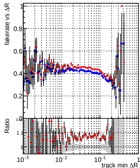
—•— DQM_mkFit_TT_retrain —•— DQM_mkFit_TTold
