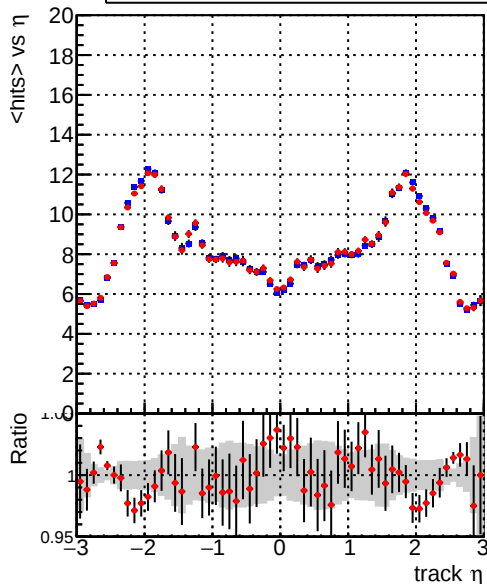
mean hits — DQM_mkFit_TT_retrain — DQM_mkFit_TTold
