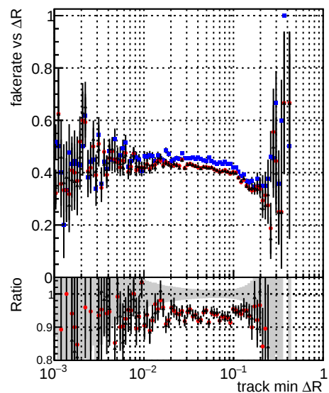
—●— DQM_mkFit5_TTold —●— DQM_mkFit_TT_retrain —●— DQM_mkFit_TT_NEWdefault_specPLeSS3
