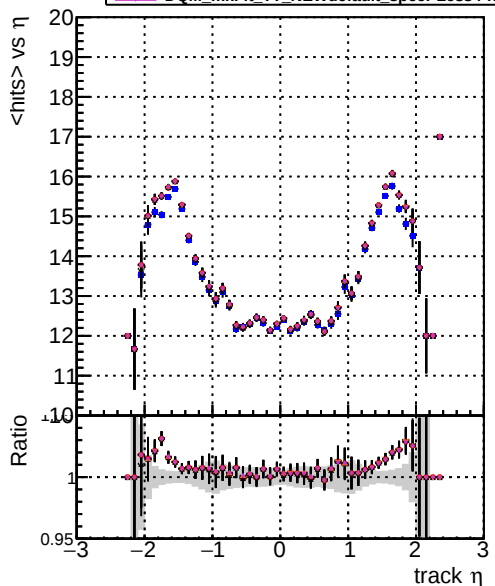
mean hits DQM mkFit TT (train-lowpt) DQM mkFit TT NEWdefault specPless1-lowpt DQM mkFit TT NEWdefault specPless2-lowpt DQM mkFit TT NEWdefault specPless3-lowpt DQM mkFit TT NEWdefault specPless4-lowpt
