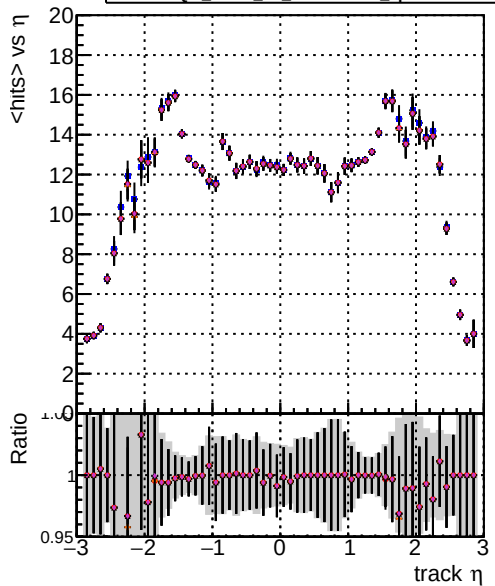
Legend: DQM mkFit TT NEWdefault specPless1-lowpt, DQM mkFit TT NEWdefault specPless2-lowpt, DQM mkFit TT NEWdefault specPless3-lowpt, DQM mkFit TT NEWdefault specPless4-lowpt mean hits
