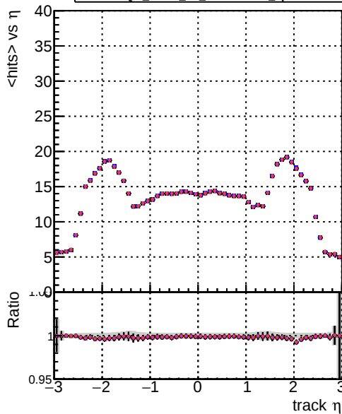
mean hits DQM mkFit TT retain_lowpt DQM mkFit TT NEWdefault specPless1_lowpt DQM mkFit TT NEWdefault specPless2_lowpt DQM mkFit TT NEWdefault specPless3_lowpt DQM mkFit TT NEWdefault specPless4_lowpt
