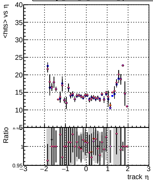
Legend: DQM mkFit TT (train-lowpt), DQM mkFit TT NEWdefault specPless1-lowpt, DQM mkFit TT NEWdefault specPless2-lowpt, DQM mkFit TT NEWdefault specPless3-lowpt, DQM mkFit TT NEWdefault specPless4-lowpt mean hits
