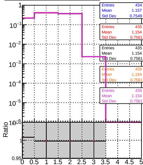
mean hit DQM mkFit TT retail-lowpt DQM mkFit TT NEWdefault specPless1-lowpt DQM mkFit TT NEWdefault specPless2-lowpt DQM mkFit TT NEWdefault specPless3-lowpt DQM mkFit TT NEWdefault specPless4-lowpt
