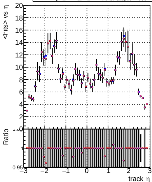
mean hits vs \eta Legend: DQM mkFit TT NEWdefault specPless1-lowpt, DQM mkFit TT NEWdefault specPless2-lowpt, DQM mkFit TT NEWdefault specPless3-lowpt, DQM mkFit TT NEWdefault specPless4-lowpt
