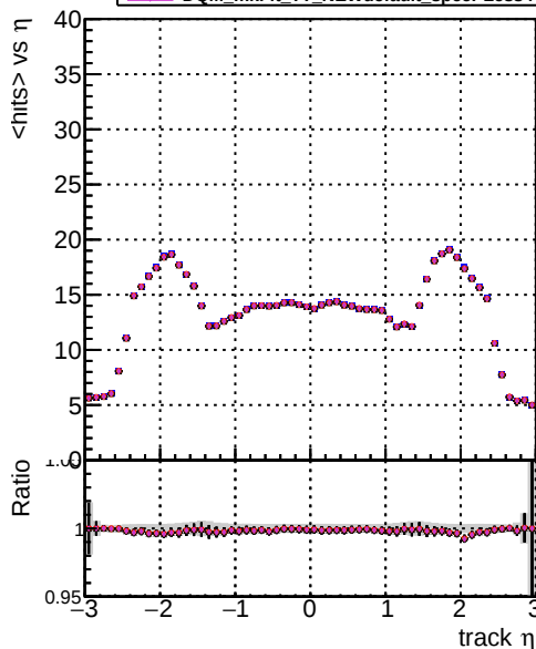
mean hits vs \eta DQM mkFit TT retain-lowpt DQM mkFit TT NEWdefault specPless1-lowpt DQM mkFit TT NEWdefault specPless2-lowpt DQM mkFit TT NEWdefault specPless3-lowpt DQM mkFit TT NEWdefault specPless4-lowpt
