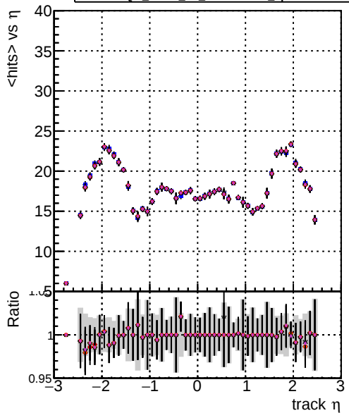
mean hits vs \eta Legend: DQM mkFit TT (train-lowpt), DQM mkFit TT NEWdefault specPless1-lowpt, DQM mkFit TT NEWdefault specPless2-lowpt, DQM mkFit TT NEWdefault specPless3-lowpt, DQM mkFit TT NEWdefault specPless4-lowpt
