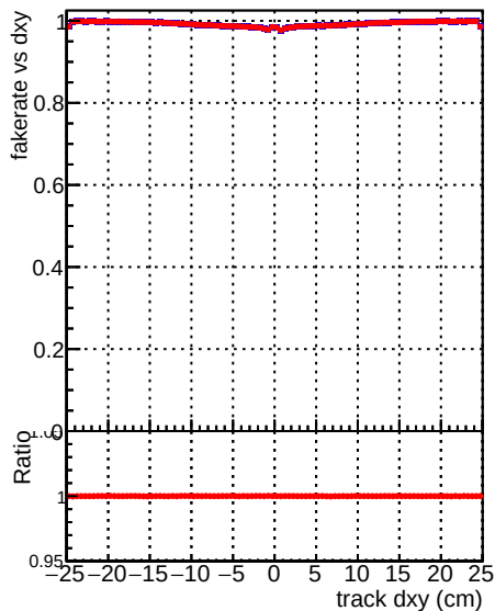
—•— DQM_mkFit_TT_retrain-lowpT —•— DQM_mkFit_TTold-lowpT
