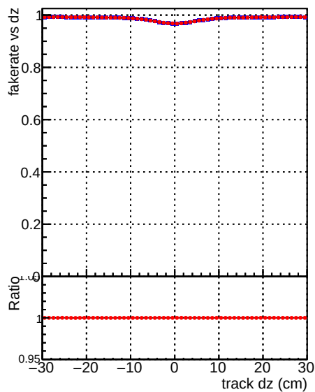
—•— DQM_mkFit_TT_retrain-lowpT —•— DQM_mkFit_TTold-lowpT
