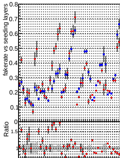
—●— DQM_mkFit_TT_retrain-lowpt —●— DQM_mkFit_TTold-lowpt
