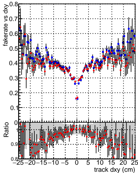
■ DQM_mkFit_TT_retrain-lowpT ● DQM_mkFit_TTold-lowpT
