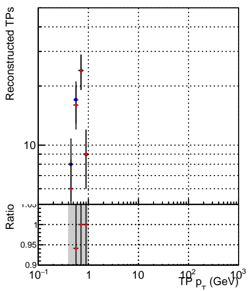
■ DQM_mkFit_TT_retrain-lowpt ● DQM_mkFit_TTold-lowpt
