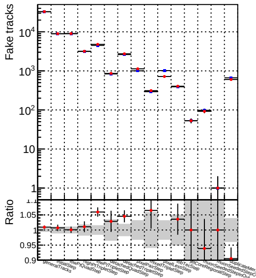
DQM_mkFit_TTold-lowpt
