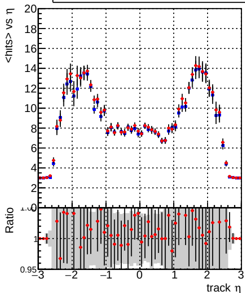
— DQM_mkFit_TT_retrain-lowpT — DQM_mkFit_TTold-lowpT mean hits
