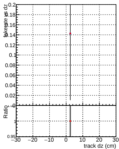
—•— DQM_mkFit_TT_retrain-lowpt —•— DQM_mkFit_TTold-lowpt
