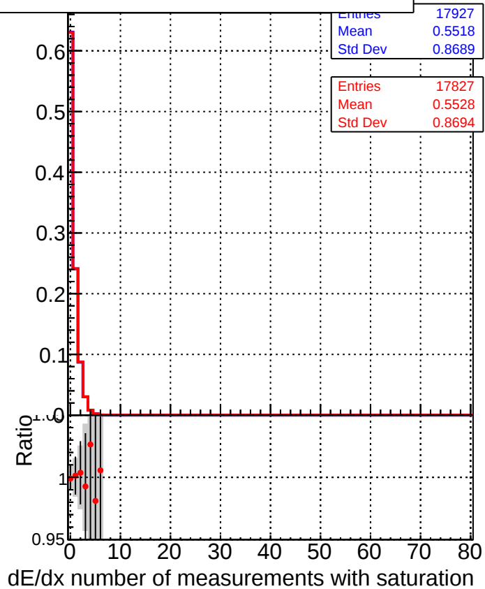
DQM_mkFit_TT_retrain-lowpt DQM_mkFit_TTold-lowpt
