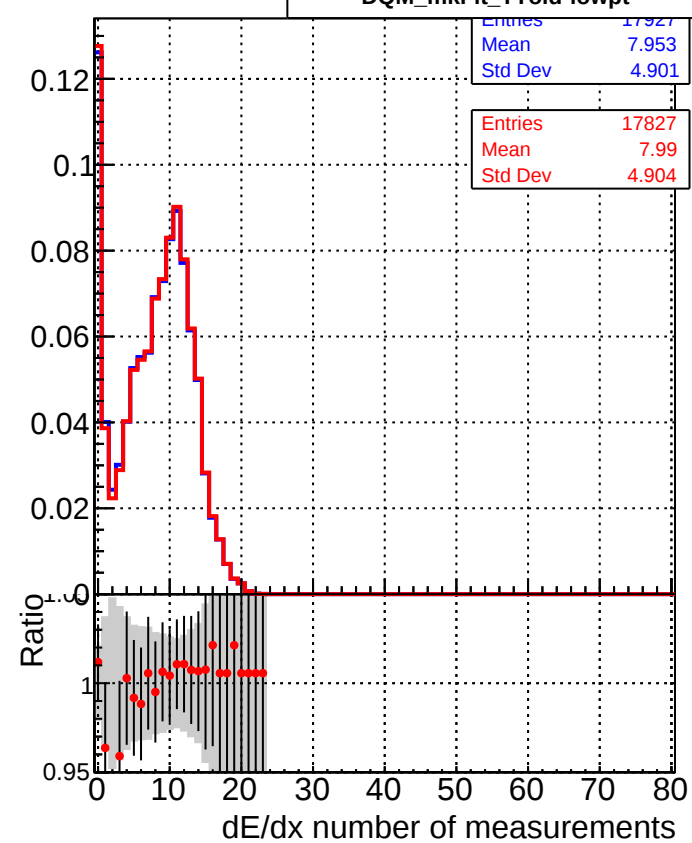
DQM_mkFit_TT_retrain-lowpt DQM_mkFit_TTold-lowpt
