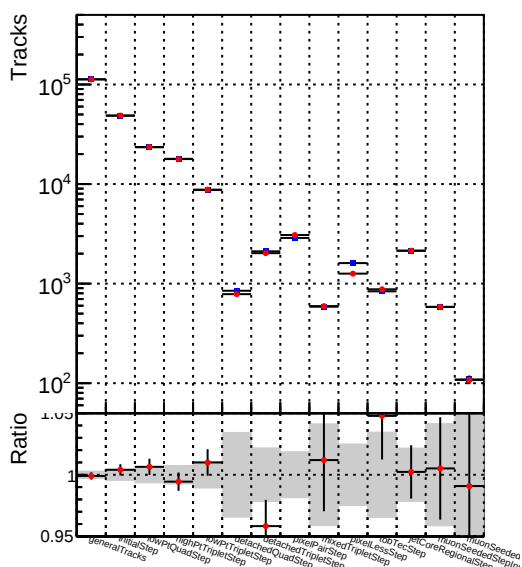
■ DQM_mkFit_TT_retrain-lowpt
