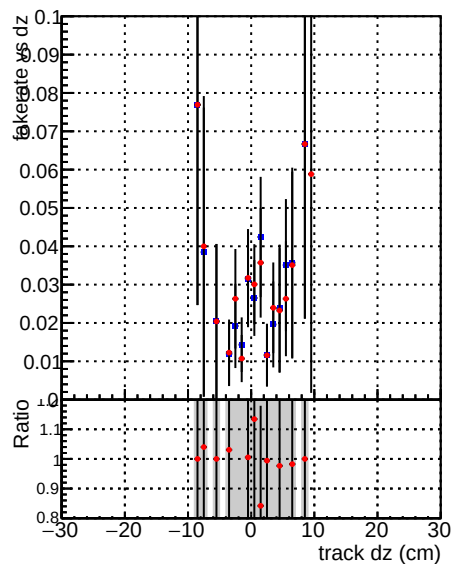
—•— DQM_mkFit_TT_retrain-lowpt —•— DQM_mkFit_TTold-lowpt
