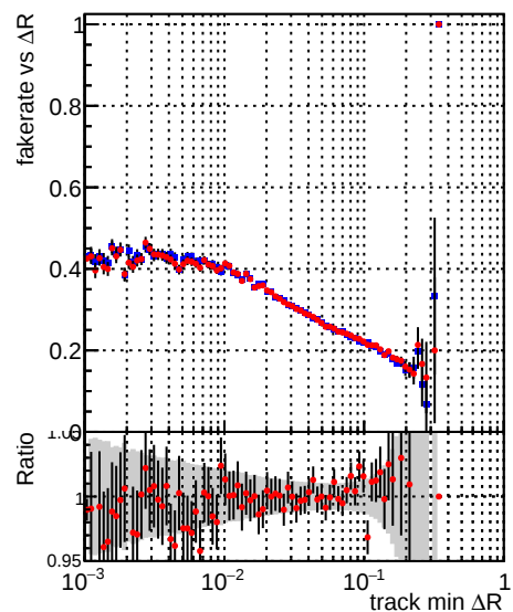
—●— DQM_mkFit_TT_retrain-lowpt —●— DQM_mkFit_TTold-lowpt
