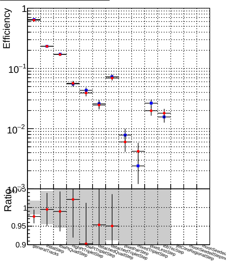
DQM_mkFit_TT_retrain-lowpt DQM_mkFit_TTold-lowpt
