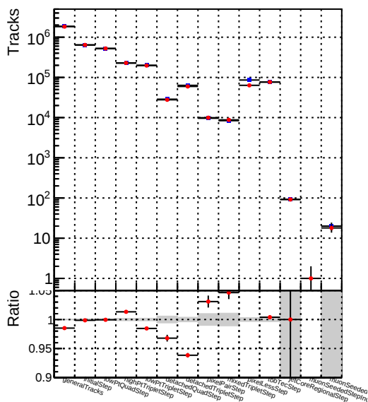
■ DQM_mkFit_TT_retrain-lowpt
