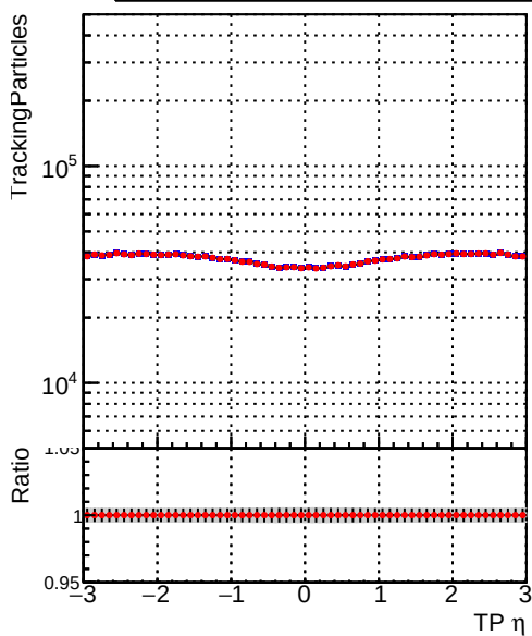
◆ DQM_mkFit_TT_retrain-lowpt ● DQM_mkFit_TTold-lowpt
