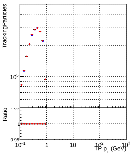
◆ DQM_mkFit_TT_retrain-lowpt ● DQM_mkFit_TTold-lowpt
