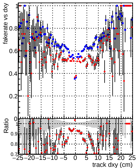
—●— DQM_mkFit_TT_retrain-lowp —●— DQM_mkFit_TTold-lowp
