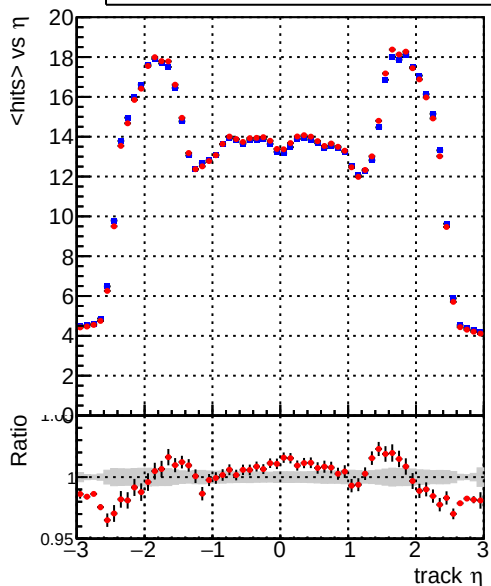
DQM_mkFit_TT_retrain-lowpt mean hits DQM_mkFit_TTold-lowpt
