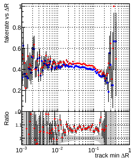
—•— DQM_mkFit_TT_retrain-lowpt —•— DQM_mkFit_TTold-lowpt
