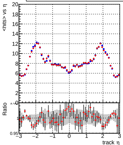
mean hits — DQM_mkFit_TT_retrain-lowpt — DQM_mkFit_TTold-lowpt
