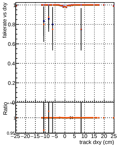
DQM mkFit5 Told lowpt DQM mkFit1 NEW default specPless3-lowpt
