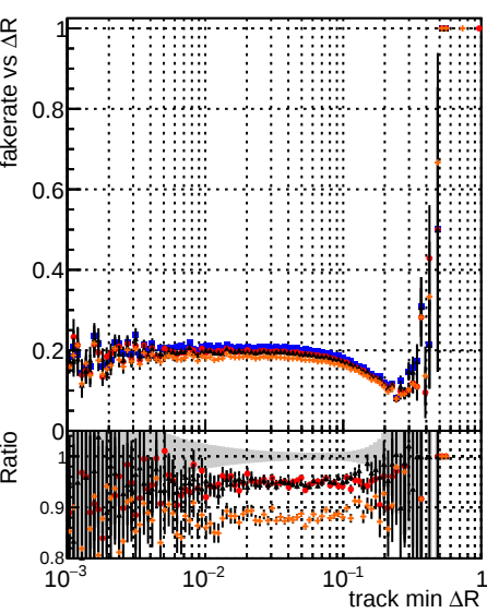
Fake rate vs \Delta R(\text{track, jet}) DQM mktFit5 Told-lowpt DQM mktFit3 Told-train-lowpt DQM mktFit1 Told-train-lowpt DQM mktFit1 NEWdefault specPLe3-lowpt
