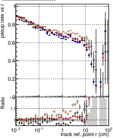
— DGM — mkFit — EIT — Told — lowpt + DGM + mkFit + EIT + Told + lowpt — DGM — mkFit — EIT — Told — lowpt — NEWDefault — specPLeas3-lowpt
