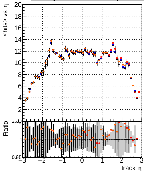
mean hit DQM_mkFit5 TTold-lowpt DQM_mkFit TT_retrain-lowpt DQM_mkFit TTold-lowpt DQM_mkFit TT_NEWdefault_specPless3-lowpt
