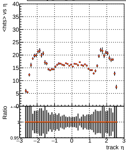
DQM_mkFit5_TTold-lowpt DQM_mkFit_TT_retrain-lowpt DQM_mkFit_TTold-lowpt DQM_mkFit_TT_NEWdefault_specPLess3-lowpt
