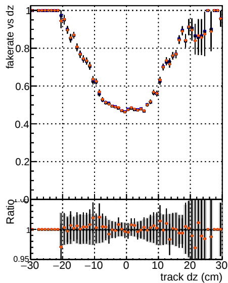
Fake rate vs dz Legend: DQM mkt TTold lowpt DQM mkt TTold lowpt DQM mkt TTold lowpt specPless3-lowpt
