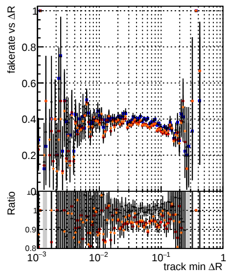
—•— DQM mkFit5 Told-lowpt —•— DQM mkFit5 Told-train-lowpt —•— DQM mkFit5 NEWdefault specPless3-lowpt
