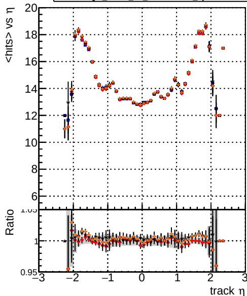
mean hits DQM_mkFit5_TTold-lowpt DQM_mkFit_TT_retrain-lowpt DQM_mkFit_TTold-lowpt DQM_mkFit_TT_NEWdefault_specPLess3-lowpt
