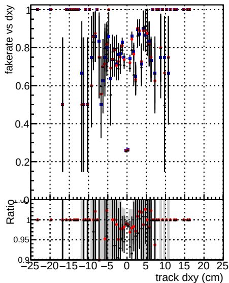
— DOM mkFit5 TTold-lowpt — DOM mkFit5 Tnew-lowpt — DOM mkFit5 TNEWdefault — DOM mkFit5 TspecPless3-lowpt
