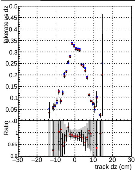
— DOM mkFit5 TTold-lowpt — DOM mkFit5 Tnew-lowpt — DOM mkFit5 TNEWdefault — DOM mkFit5 TspecPless3-lowpt
