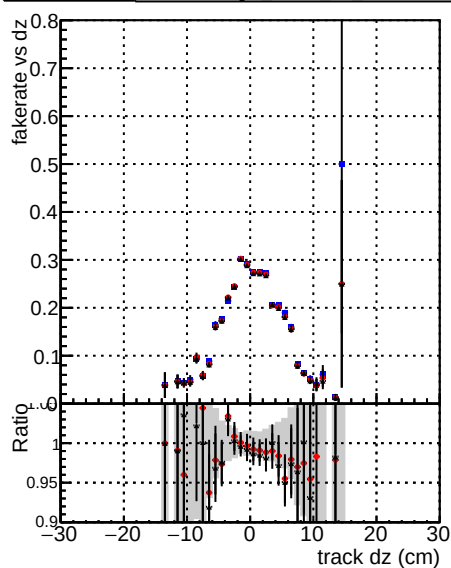
— DOM mkFit5 TTold-lowpt — DOM mkFit5 Ttrain-lowpt — DOM mkFit5 TTNEWdefault specPless3-lowpt
