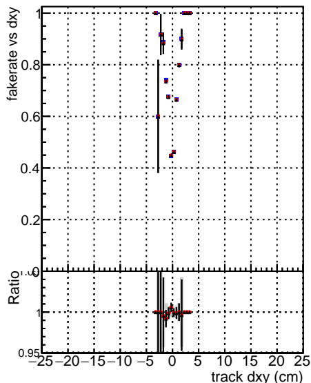
— DGM mkFit5 TTold-lowpt — DGM mkFit TTretain-lowpt — DGM mkFit TTNEWdefault specPless3-lowpt
