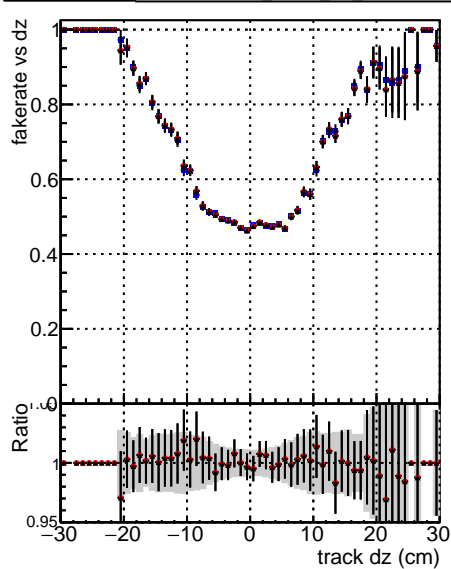
— DGM mkFit5 TTold-lowpt — DGM mkFit TTretain-lowpt — DGM mkFit TTNEWdefault specPless3-lowpt
