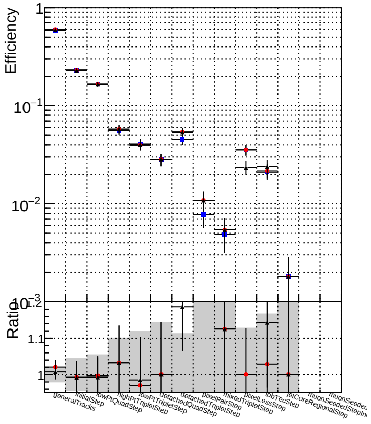
DQM_mkFit5_TTold-lowpt DQM_mkFit_TT_retrain-lowpt DQM_mkFit_TT_NEWdefault_specPLess3-lowpt
