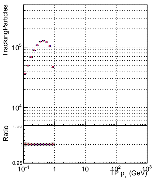
N of sim —●— DQM mkFit Ximinus NO PU NEWdefault spec Less3 —●— DQM mkFit Ximinus NO PU NEWdefault spec Less3 —●— DQM mkFit Ximinus NO PU NEWdefault spec Less3 —●— DQM mkFit Ximinus NO PU NEWdefault spec Less3
