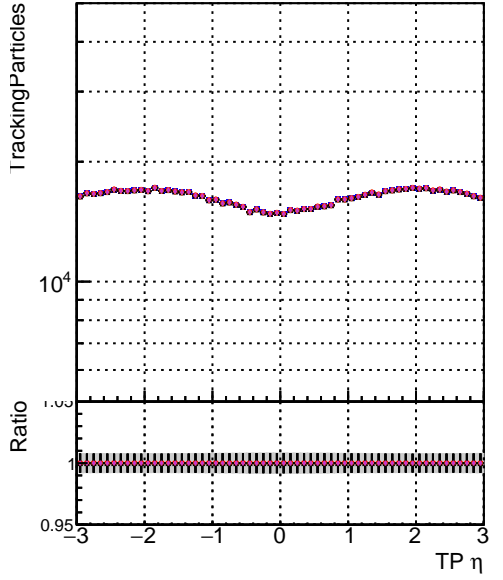
N of sim DQM mkFit Ximinus NO PU NEWdefault spec Less3 Less3 Less3 Less3 + + + + + + + + + +
