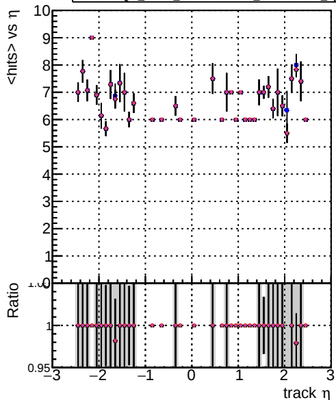
Legend: DQM mkFit XiminusNOPU NEWdefault specPless1, DQM mkFit XiminusNOPU NEWdefault specPless3, DQM mkFit XiminusNOPU NEWdefault specPless4 mean hits
