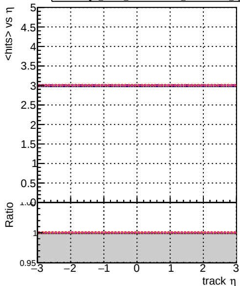
Legend: DQM mkFit XiminusNOPU NEWdefault specPless1, DQM mkFit XiminusNOPU NEWdefault specPless3, DQM mkFit XiminusNOPU NEWdefault specPless4 mean hit
