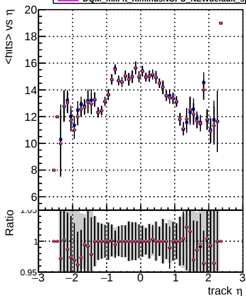
Legend: DQM mkFit XiminusNOPU NEWdefault specPless1, DQM mkFit XiminusNOPU NEWdefault specPless2, DQM mkFit XiminusNOPU NEWdefault specPless3, DQM mkFit XiminusNOPU NEWdefault specPless4
