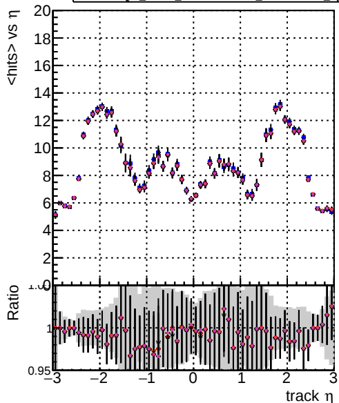
Legend: DQM mkFit XiminusNOBU NEWdefault specPless1, DQM mkFit XiminusNOBU NEWdefault specPless2, DQM mkFit XiminusNOBU NEWdefault specPless3, DQM mkFit XiminusNOBU NEWdefault specPless4 mean hit
