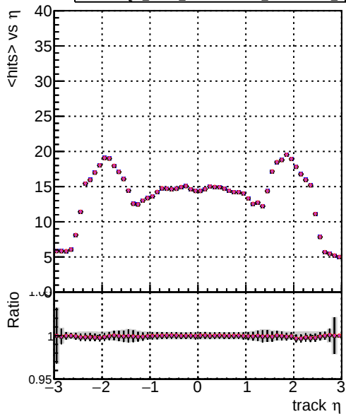
Legend: DQM mkFit XiminusNOPU NEWdefault specPless1, DQM mkFit XiminusNOPU NEWdefault specPless2, DQM mkFit XiminusNOPU NEWdefault specPless3, DQM mkFit XiminusNOPU NEWdefault specPless4 mean hit
