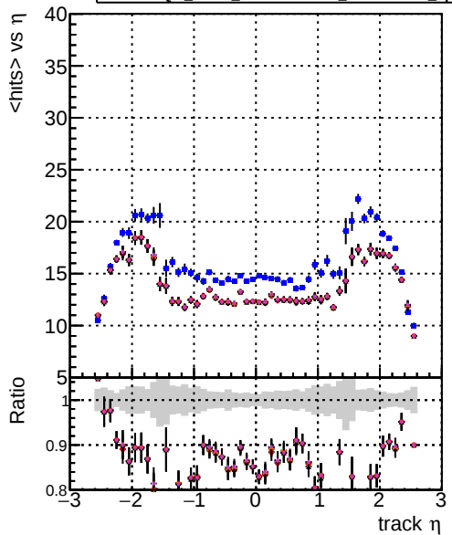
Legend: DQM mkFit XiminusNOBU NEWdefault specPless1, DQM mkFit XiminusNOBU NEWdefault specPless3, DQM mkFit XiminusNOBU NEWdefault specPless4 mean hit
