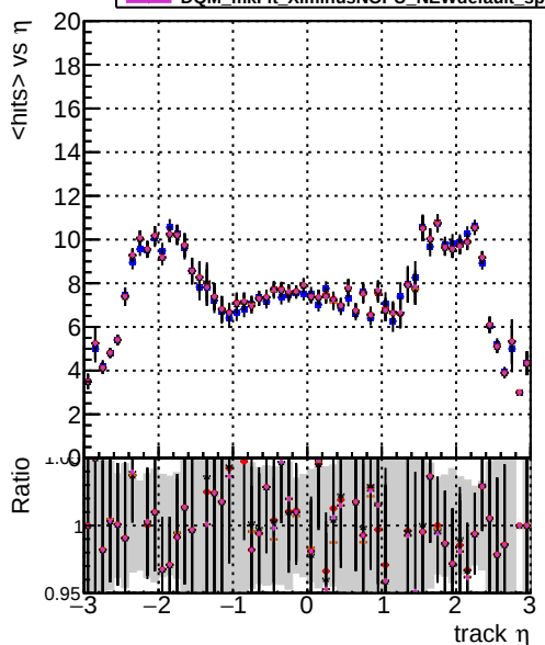
mean hit DQM mkFit XiminusNOPU NEWdefault specPless1 DQM mkFit XiminusNOPU NEWdefault specPless3 DQM mkFit XiminusNOPU NEWdefault specPless4
